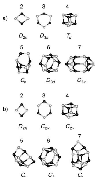
Abbildung 1. Stabile Strukturen von a) neutralen (\text{MgO})_n^- und b) kationischen (\text{MgO})_n^+ -Clustern mit n=2-7 (schwarz: Mg, weiß: O).
